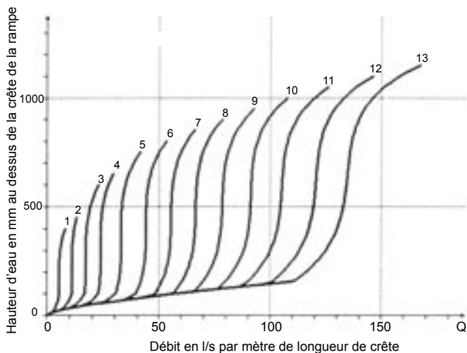
Fig. 4 : Diagramme des courbes de débits.
