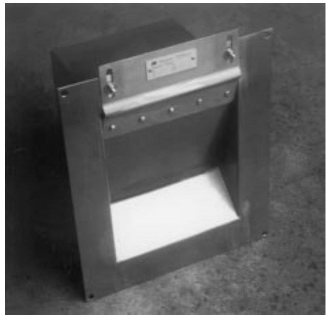
Fig. 5 : Construction spéciale d'un déversoir UFT- FluidClari en version compacte pour fixation par chevilles. Cet appareil est pré-réglé en usine sur le débit de déversement.
