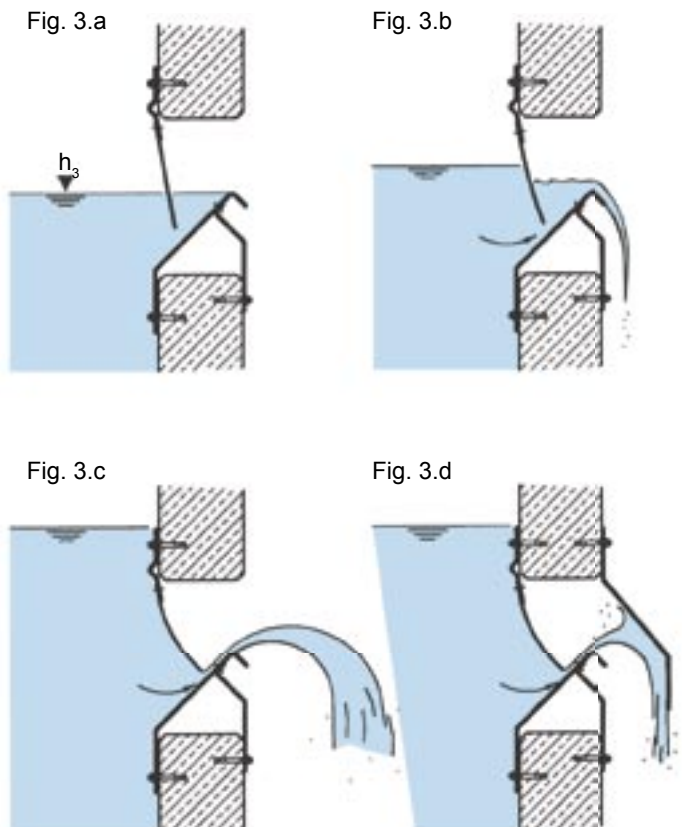
Fig. 3 : Fonctionnement du déversoir UFT-FluidClari.
