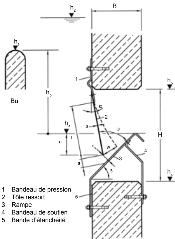
Fig. 2 : Construction du déversoir UFT-FluidClari.
