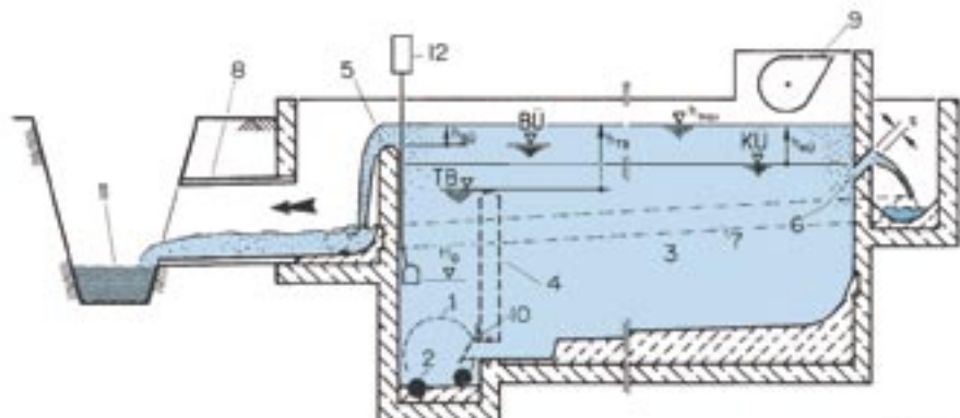
Fig. 1 : Coupe en long d'un bassin de type transit classique avec fente déversoir de traitement conventionnelle.
