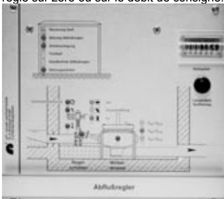
Fig. 2 : Synoptique du régulateur vortex UFT-FluidVortex-E
