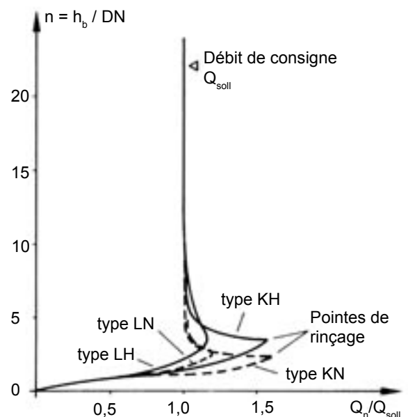
Fig. 3 : Courbes de débits, adimensionnelles du régulateur vortex UFT-FluidVortex-E.
