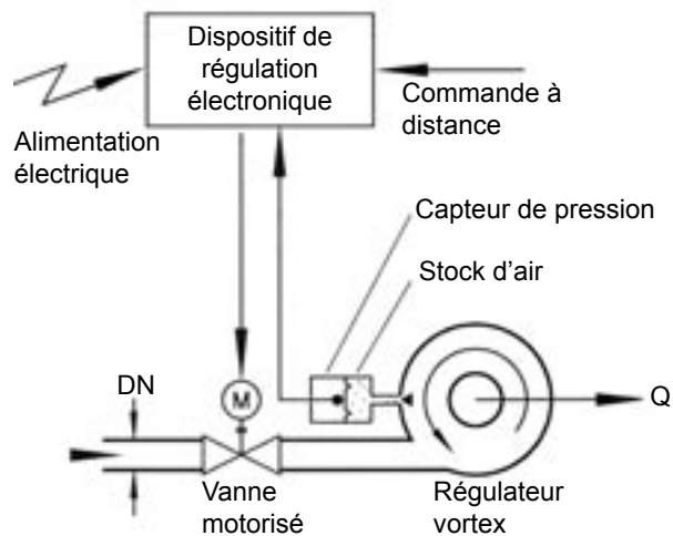
Fig. 1 : Principe et composition du circuit de régulation UFT-FluidVortex-E
