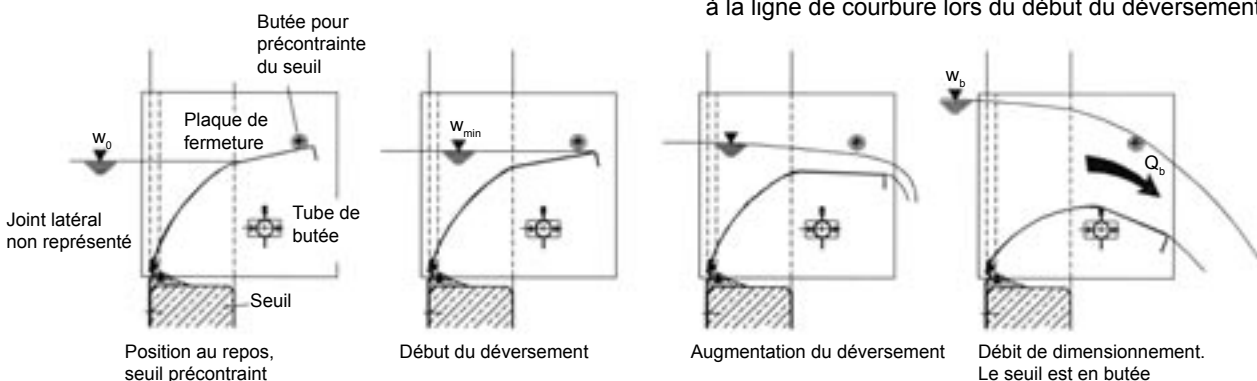
Fig. 2 : Différentes phases de travail du seuil souple UFT-FluidBend.
