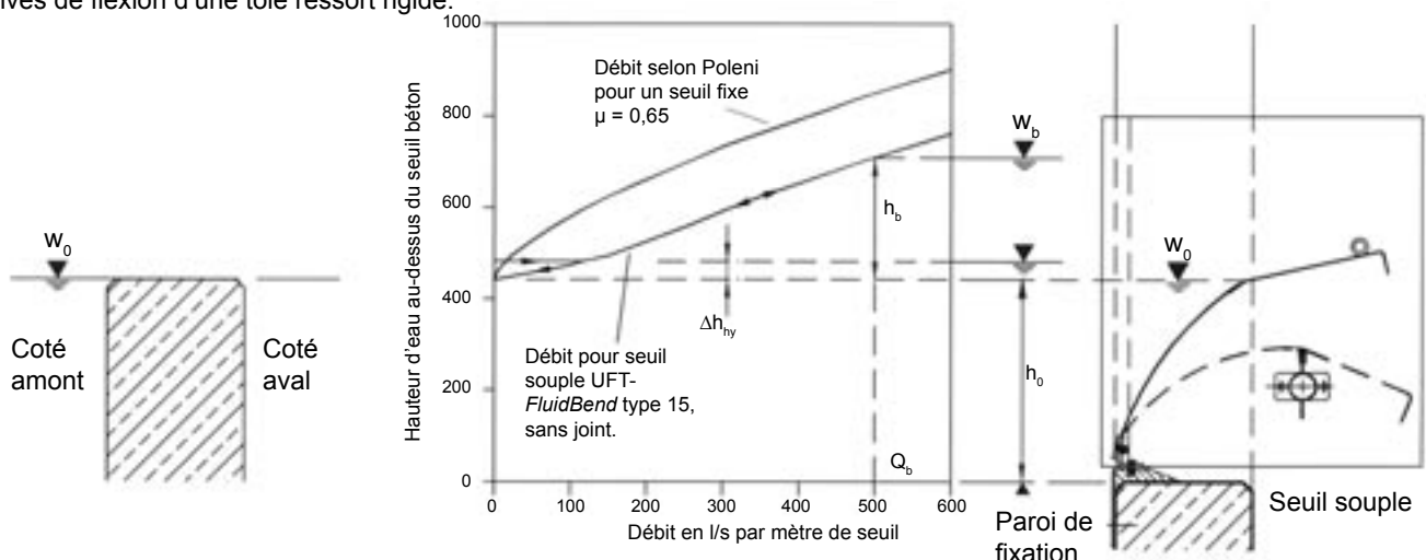
Fig. 3 : Diagramme des débits d'un seuil souple UFT-FluidBend en comparaison à un seuil fixe.
