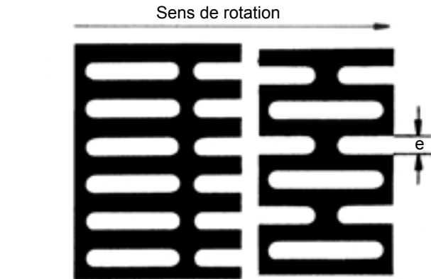
Fig. 1 : Tôle perforée en acier inoxydable avec fentes de largeur e , percements parallèles et décalés.
