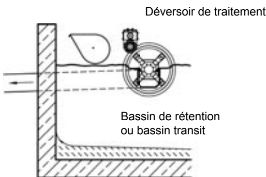
Fig. 2 : Différentes possibilités d'implantation du tamis filtre.
